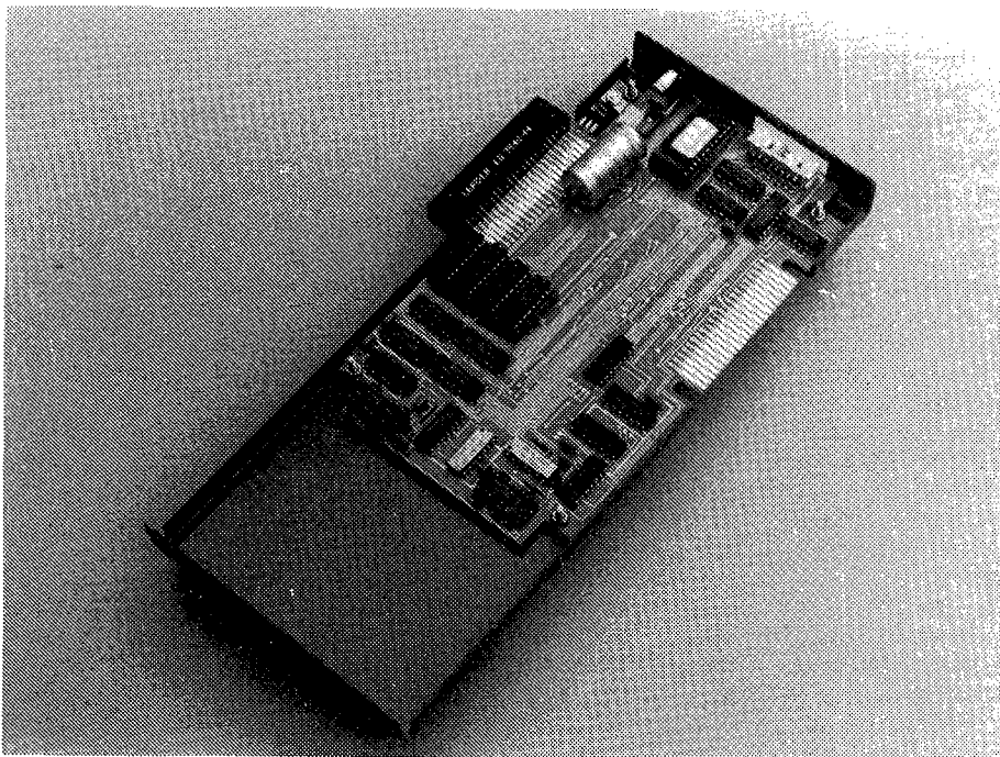
Der innere Aufbau der 128K-Erweiterung
