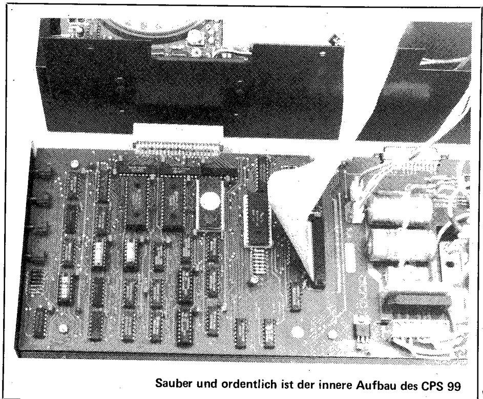
Das CPS 99 angeschlossen am TI 99/4A
